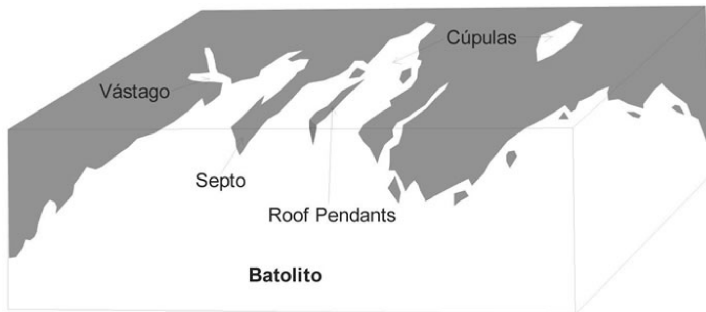
Fig. 5-7. Esquema idealizado del desarrollo de un batolito.
