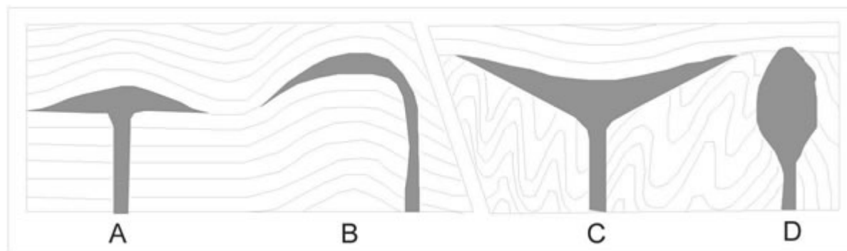
Figura 5-1. Formas de cuerpos plutónicos. A- Lacolito. B- Facolito. C- Lopolito. D- Stock (redibujado de Wimenauer, 1985).
