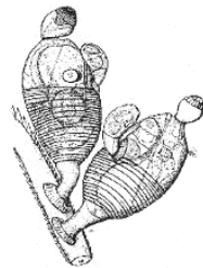
Cyclophora
